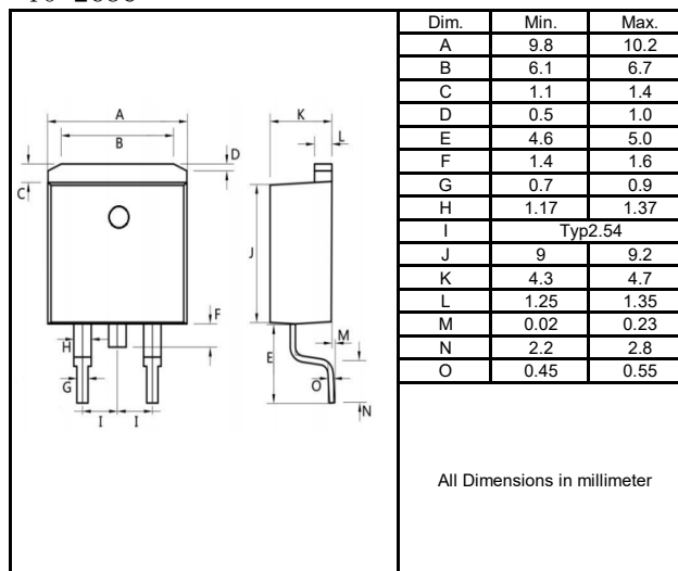
TO-263C
